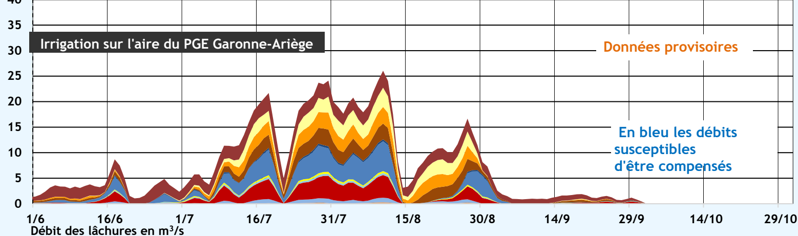
Cumuls en m³/s des débits estimés des prélèvements pour l'irrigation (eau de surface, nappe et ventilation canaux) Source modélisation E-tiage Sméag-Eaucéa
